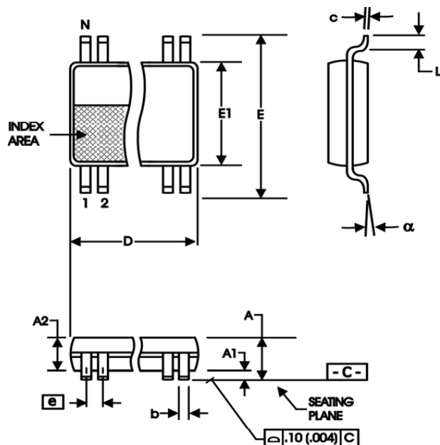
209 mil SSOP
